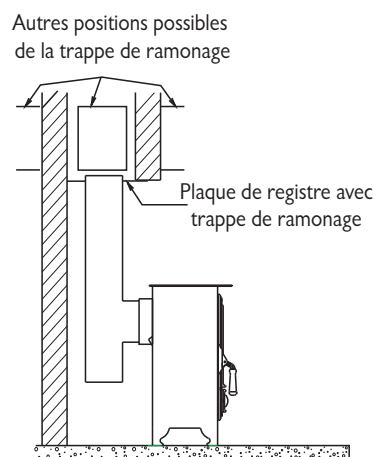
Fig. 6. Plaque de registre horizontale avec branchement de conduit de fumée par l'arrière
