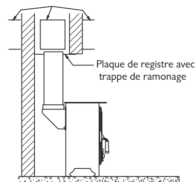
Fig. 8. Plaque de registre horizontale avec adaptateur arrière vertical en option
