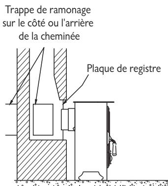
Fig. 5. Plaque de registre verticale avec cheminée maçonnée
