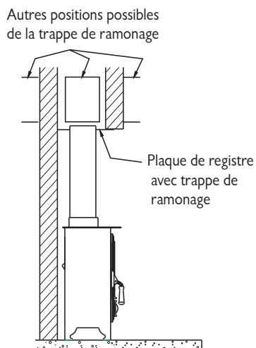
Fig. 7. Plaque de registre horizontale avec branchement de conduit de fumée vers le haut
